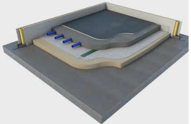
Isolation acoustique avec TRAMICHAPE FIBRE + FILM sur PU avec chauffage hydraulique
